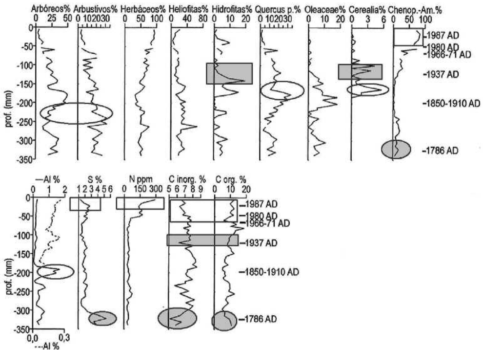
GRÁFICO 1 Registro polínico y geoquímico correspondiente a los últimos 300 años según sondeos realizados en el Parque Nacional de las Tablas de Daimiel
