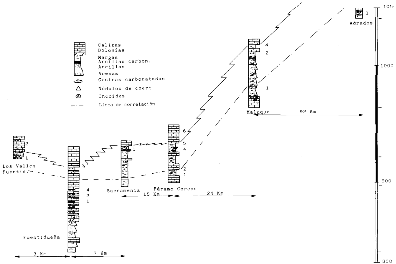
Figura 2. Correlación de las diferentes secciones.
