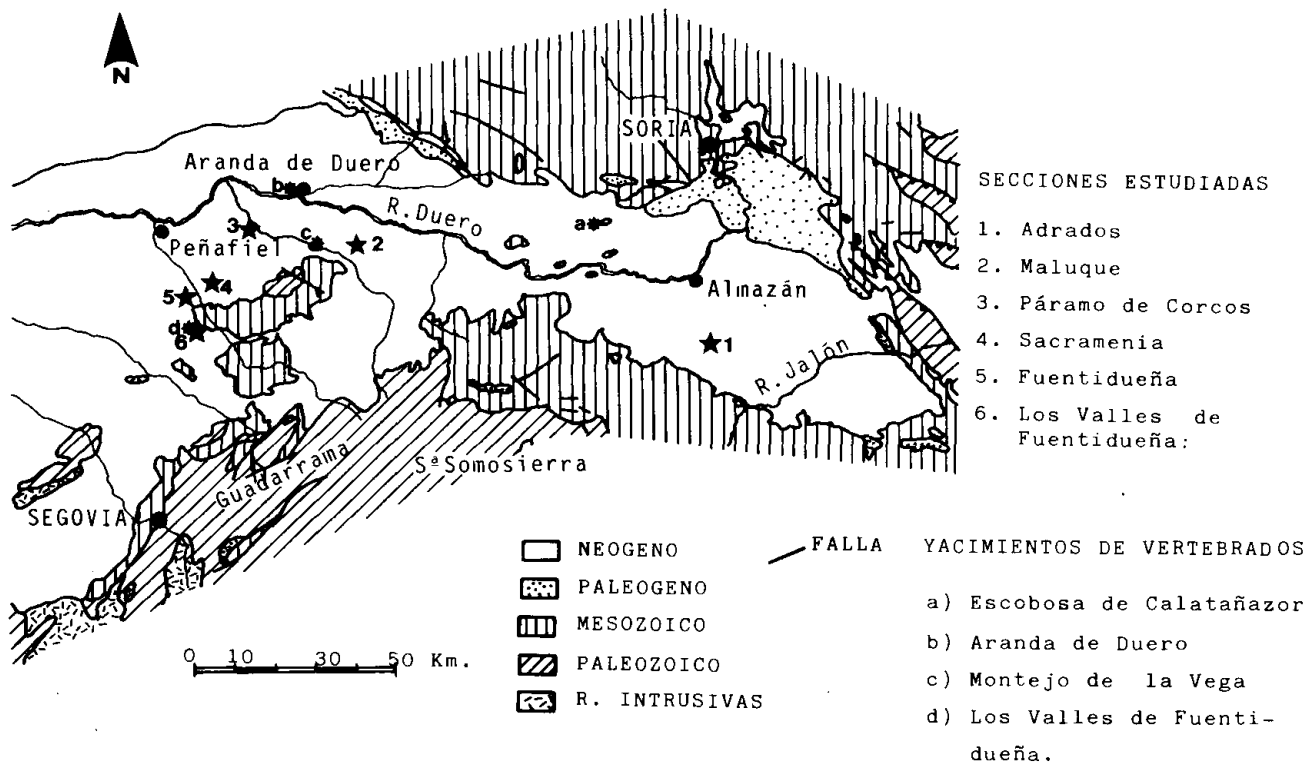
Figura 1. Esquema geológico, localización de las secciones estudiadas y de los yacimientos de vertebrados más importantes.
