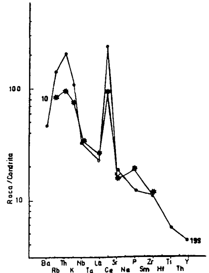
Fig. 6.—Perfiles normalizados de los elementos menores respecto a condritas.
