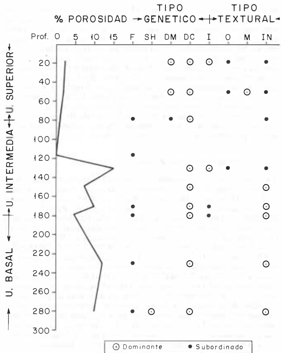
FIG. 6.—Tipos dominantes de porosidad secundaria según los criterios SCHMIDT y McDONALD (1979b) en el sondeo n.º 1 de Albarracín. F=Fract. SH=Retracción; DM=Disolución material sedimentario; DC=Disolución del cemento; I=Intergranular; O=Poros agrandados; M=Móldica; IN=Intraco-tuyente.
