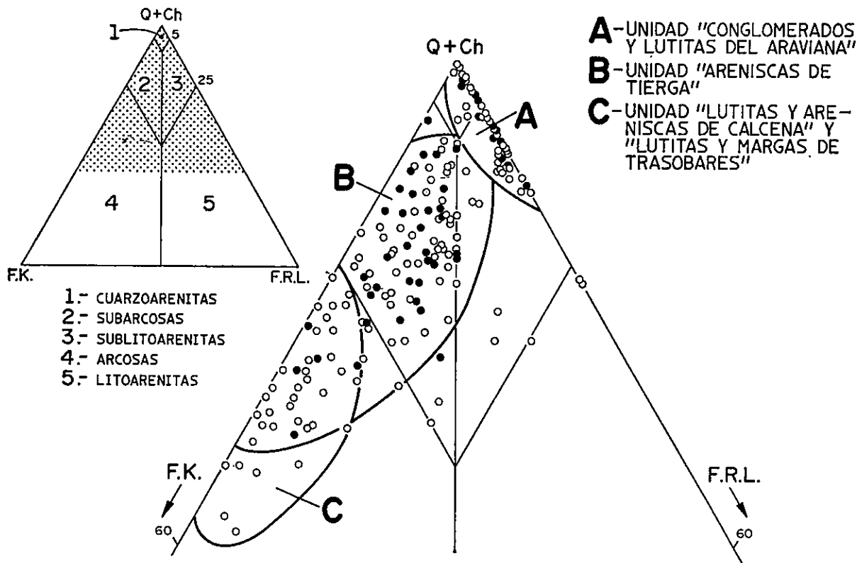
Fig. 5.—Composición general de las areniscas del Grupo Detrítico en un diagrama de Pettijohn et al. (1973). Los signos rellenos pertenecen a grauvacas (> 15% en matriz).
