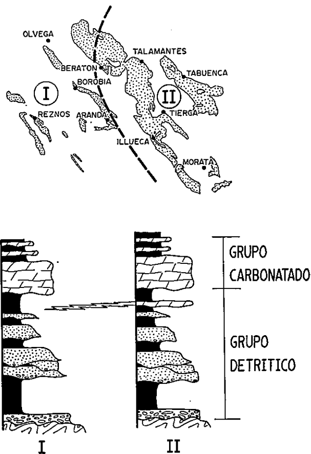
Fig. 2.—Distribución espacial de los litotipos ibérico (I) y mediterráneo (II) del Triás en el borde norte de la rama aragonesa, con la nomenclatura litoestratigráfica empleada en este trabajo.
