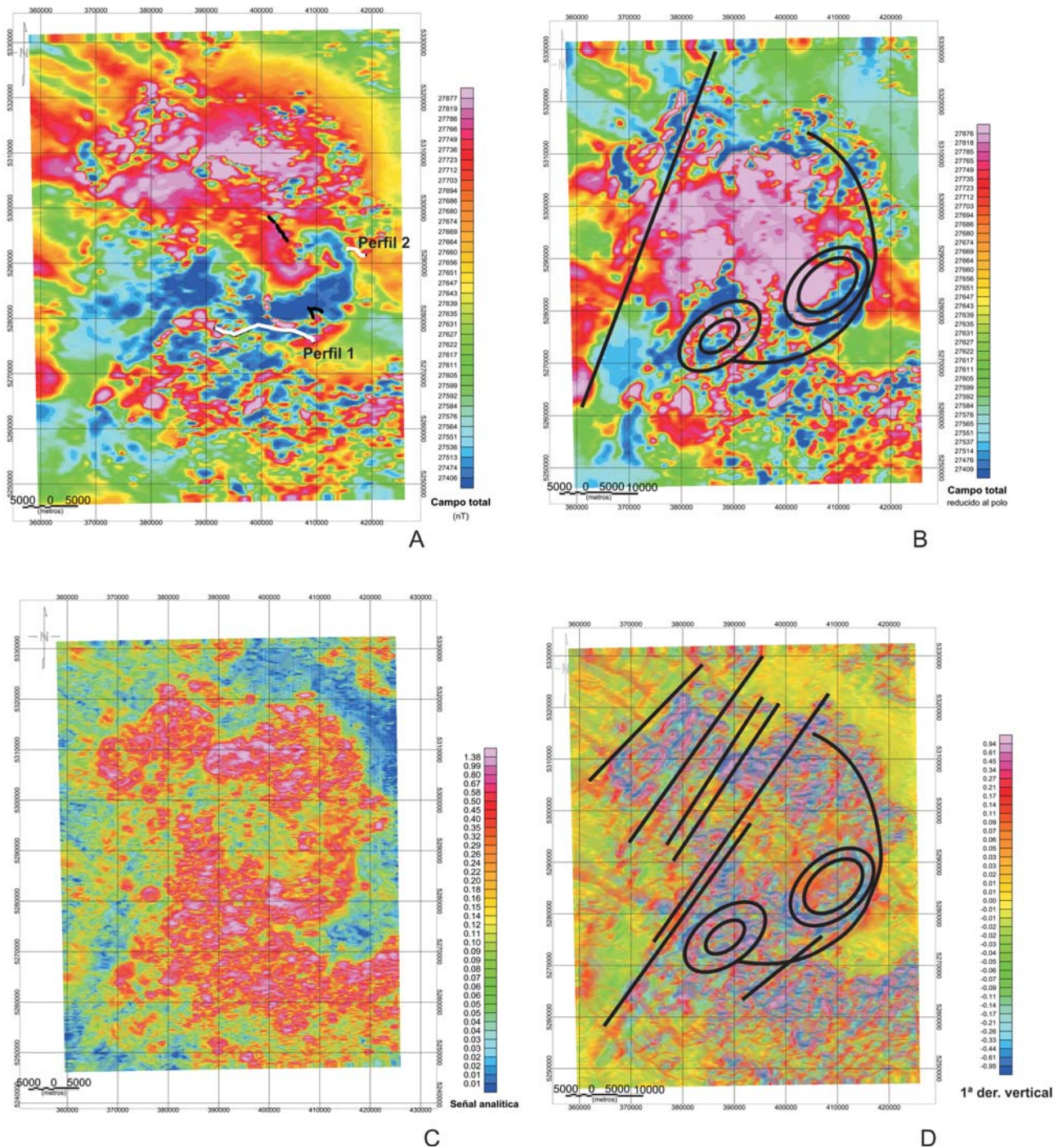
Figura 4. Mapas magnéticos de la caldera de Piedra Parada. A) Campo magnético total y situación de los perfiles magnéticos. B) Mapa del campo magnético total reducido al polo. C) Mapa de señal analítica. D) 1ª derivada vertical del campo reducido al polo. En los mapas B y D se han indicado las estructuras magnéticas más significativas.
