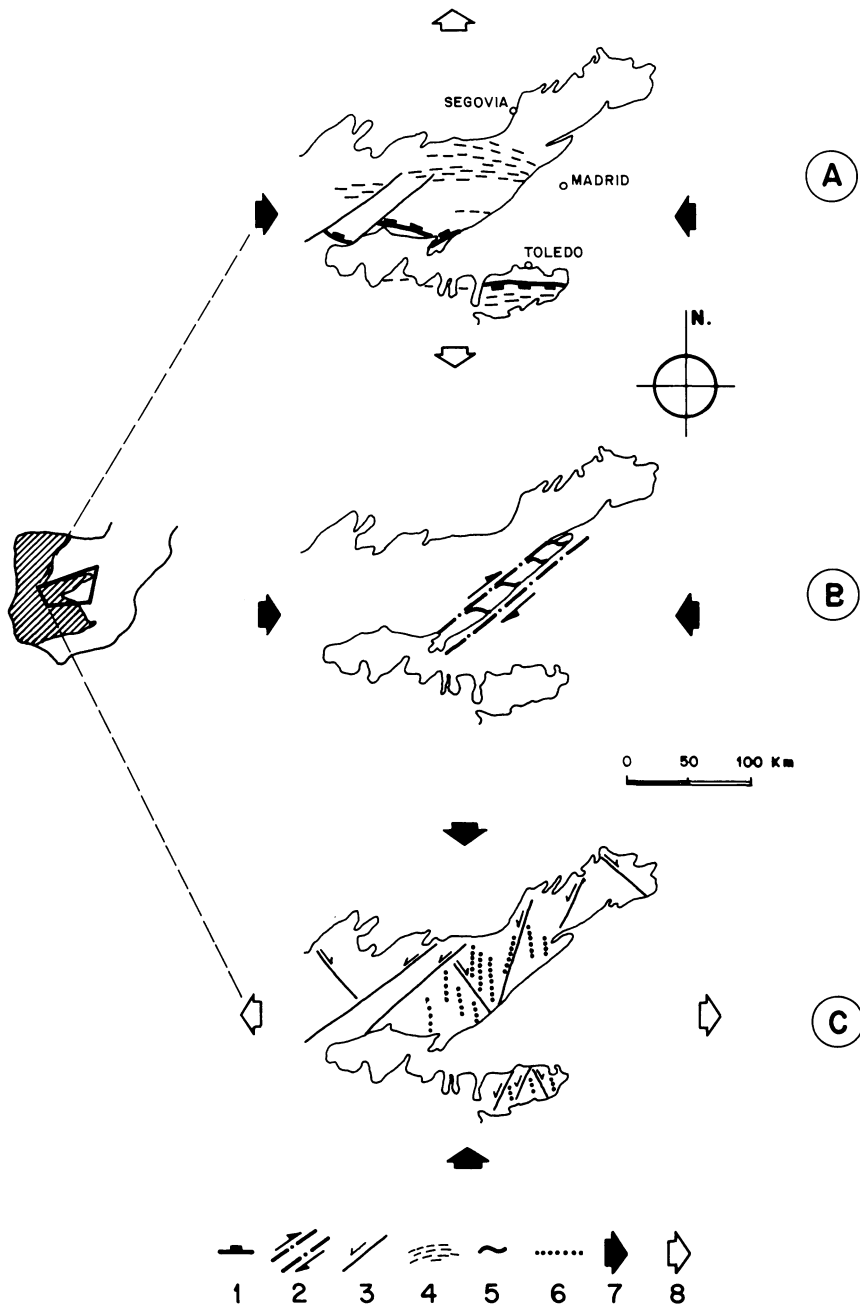
Fig. 1 Sistemas filonianos y estados de esfuerzos asociados en el centro peninsular durante los tres episodios tectónicos tardihercénicos. A) Episodio dúctil extensional. B) Episodio dúctil/frágil transcurrente. C) Episodio frágil transcurrente. 1: superficies de detachment; 2: corredor transcurrente dextral; 3: fallas frágiles; 4: diques de pórfido y aplita; 5: filones de baritina; 6: diques de cuarzo, diabasa, y lamprófito; 7: dirección de compresión; 8: dirección de extensión.
