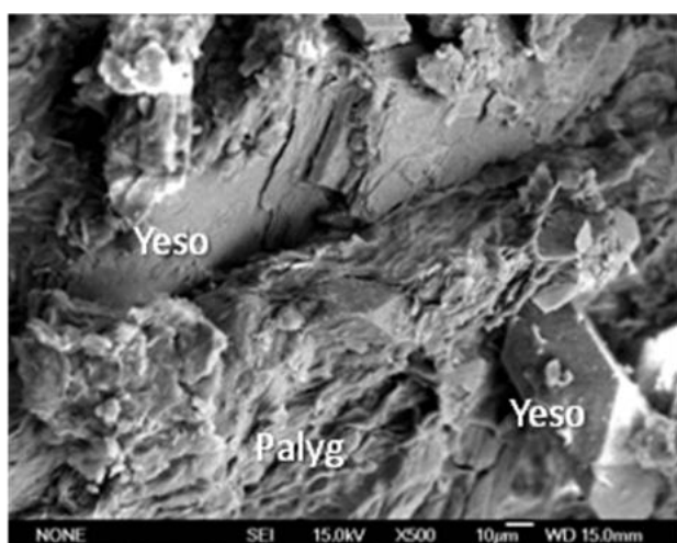
Fig.2 Muestra 110-112. Cristales de yeso rodeados de Palygorskita.
