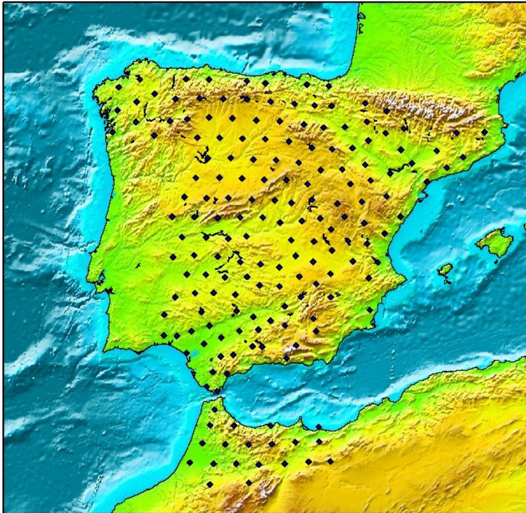
FIGURA 1. Distribución de las estaciones sísmicas planeadas para en España y norte de Marruecos de Iberarray. Además de esta distribución hay que incluir las estaciones sísmicas, de banda ancha, de redes locales, regionales y nacionales de los diferentes grupos que integran TOPOIBERIA.
