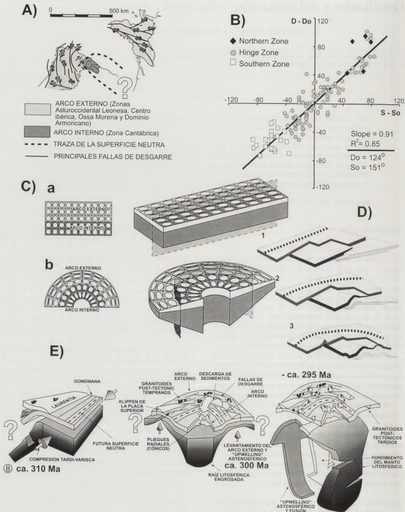
FIGURA 1. A) Esquema geológico del CVOE; B) Desviaciones de la declinación respecto a la dirección de referencia (Modificado de Weil et al., 2001); C) Esquema ilustrando el mecanismo de deformación longitudinal tangencial; D) Esquema del desarrollo de pliegues cónicos los mantos más occidentales de la Zona Cantábrica; y E) Esquema ilustrativo de la evolución tectónica propuesta para el caso de una delaminación litosférica causada por la generación de un orocinal.
