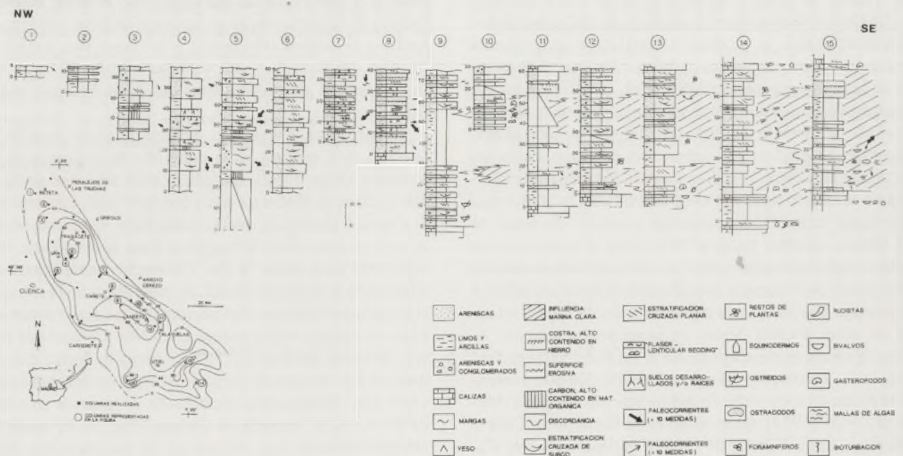
FIGURA 2: Situación del área estudiada, mapa de isopacas del Mb. El Bural y correlación de columnas seleccionadas.
