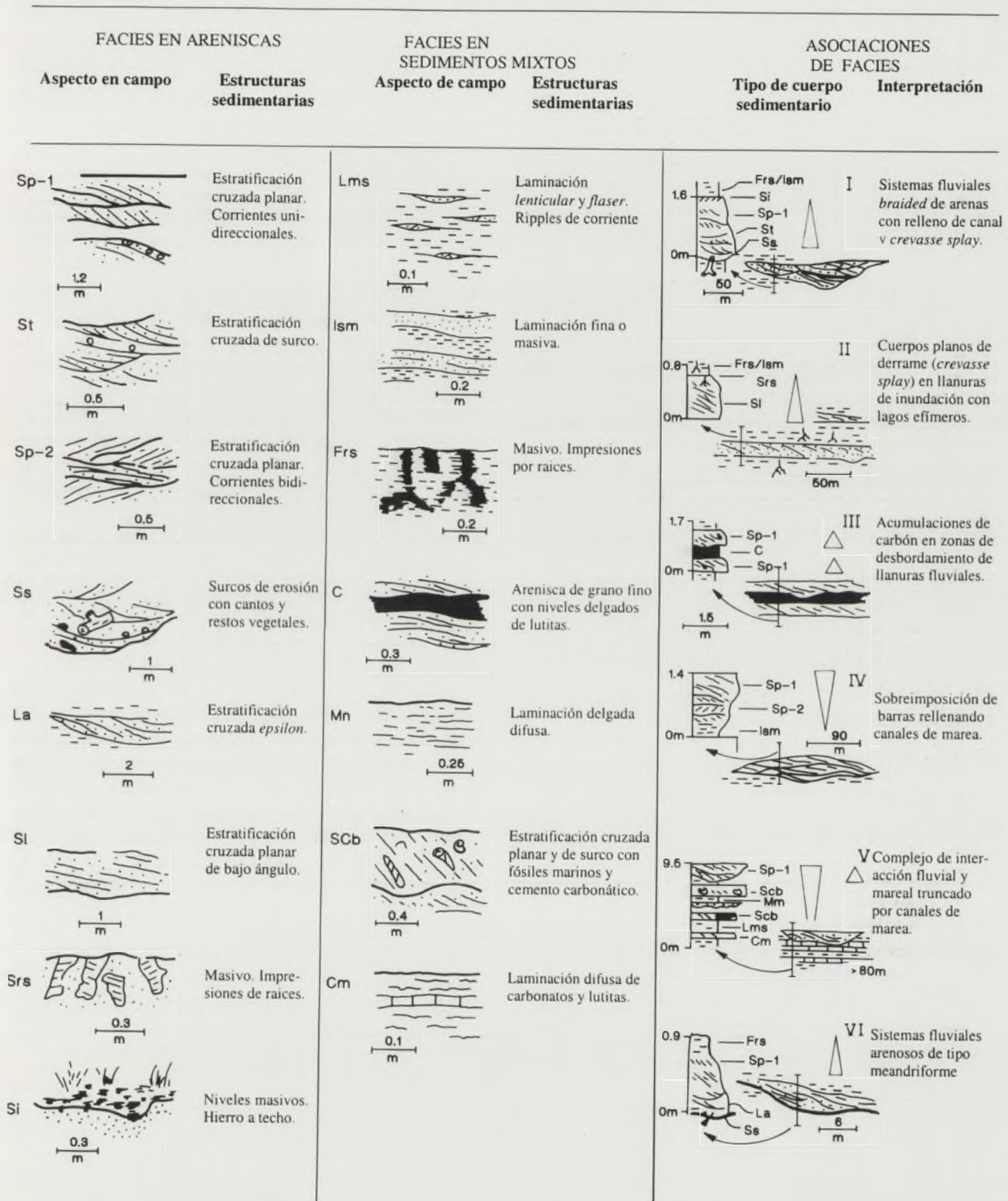
FIGURA 3: Facies y asociaciones de facies diferenciadas en el Mb. El Buralgal.
