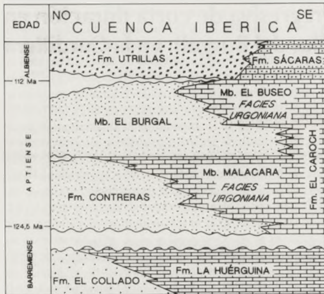
FIGURA 1: Cronoestratigrafía de la Cuenca Ibérica Suroccidental según Vilas et al. (1982) para el intervalo Barremiense-Aptiense, modificado a partir de los datos del área estudiada.
